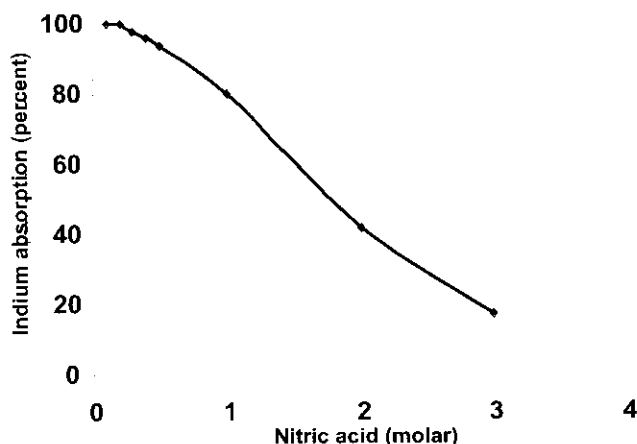
شکل ۱- نمودار تغییرات میزان جذب ایندیوم بر اثر تغییر غلظت اسیدنیتریک (سرعت جریان 1 میلی‌لیتر بر دقیقه، ستون حاوی 4 گرم رزین با ابعاد 200 \times 16 میلی‌متر).
