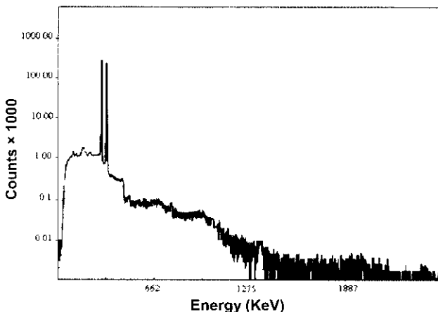
شکل ۲- طیف گامای ^{113m}\text{In} پس از عملیات جداسازی.
