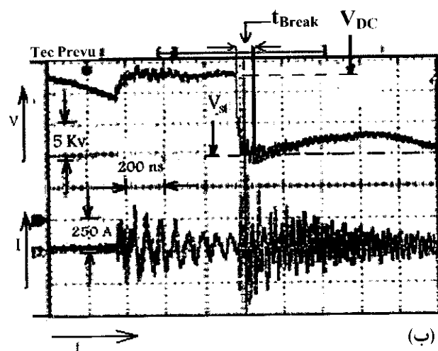
شکل ۵- تغییرات زمانی ولتاژ کلید و جریان عبوری از آن در مقیاسهای زمانی مختلف الف- مقیاس زمانی ۲۰ میلی‌ثانیه، ب- مقیاس زمانی ۲۰۰ نانو ثانیه. رفتارهای زمانی V و I برتریب در تصاویر بالا و پایین نشان داده شده‌اند.
