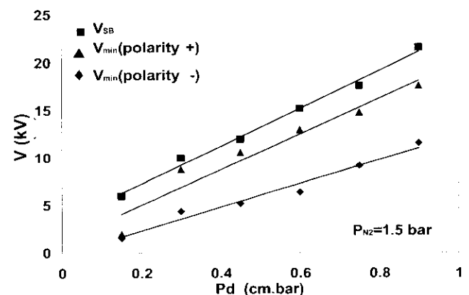
شکل ۴- تغییر ولتاژ شکست کلید تریگاترون بر حسب حاصلضرب فشار، p، و فاصله الکترودها، d.
