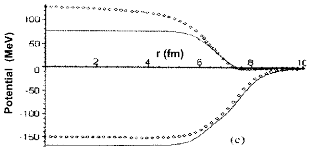
شکل ۲- قسمتهای حقیقی و موهومی پتانسیل ایتیکی موضعی برای ^{208}_{82}Pb در انرژیهای a: 162 MeV, b: 180 MeV, c: 291 MeV.
