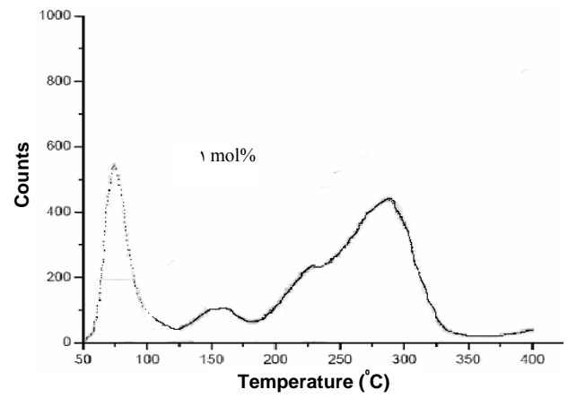
شکل ۴- منحنی درخشش ترکیب کلسیم فلورید با ۱ درصد مولی از Dy، به دست آمده با استفاده از دستگاه TLD-خوان. قله‌ها تقریباً در ۱۵۵، ۲۲۵ و ۲۹۵°C مشاهده شده‌اند. [آهنگ گرمایش ۱۰، ۱۰°C/S، ۱۰ ثانیه در ۱۰۰°C].
