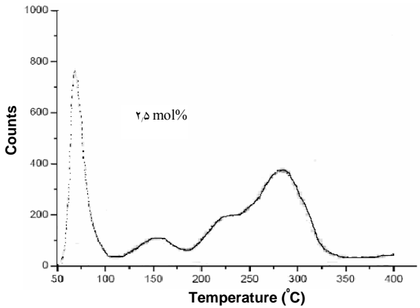
شکل ۷- منحنی درخشش ترکیب کلسیم فلورید با ۲٫۵ درصد مولی از Dy، به دست آمده با استفاده از دستگاه TLD-خوان. دماهای نظیر قله‌ها عبارت‌اند از تقریباً ۱۵۵، ۲۲۵ و ۲۹۵°C. [آهنگ گرمایش ۱۰، ۱۰°C/S، ۱۰ ثانیه در ۱۰۰°C].
