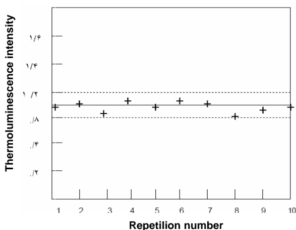
شکل ۱۱- تغییرات شدت نوردهی به صورت تابعی از عملیات پخت تکراری (انحراف میانگین ۸٪ است).
