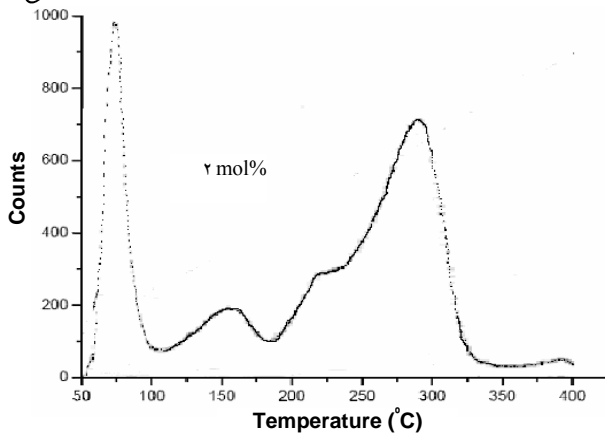
شکل ۶- منحنی درخشش ترکیب کلسیم فلورید با ۲ درصد مولی از Dy، به دست آمده با استفاده از دستگاه TLD-خوان. قله‌ها تقریباً در دماهای ۱۵۵، ۲۲۵ و ۲۹۵°C مشاهده می‌شوند. [آهنگ گرمایش ۱۰، ۱۰°C/S، ۱۰ ثانیه در ۱۰۰°C].
