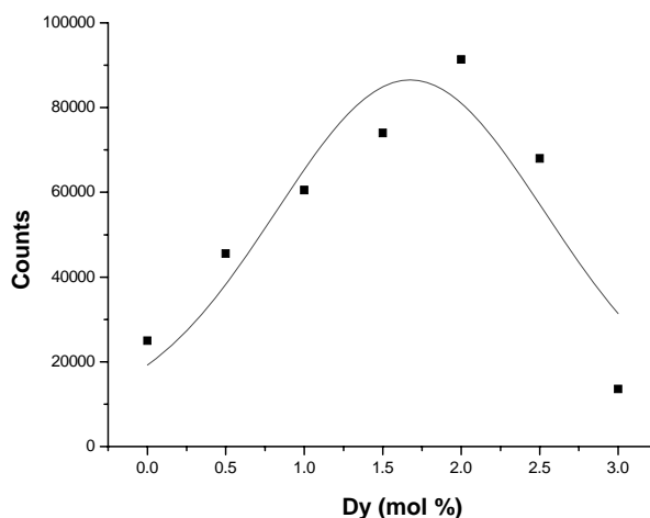
شکل ۹- تغییر شدت نوردهی با تغییر غلظت Dy.
