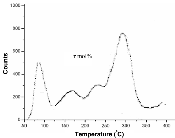
شکل ۸- منحنی درخشش ترکیب کلسیم فلورید با ۳ درصد مولی از Dy، به دست آمده با استفاده از دستگاه TLD-خوان. دماهای متناظر با قله‌ها تقریباً ۱۵۵، ۲۲۵ و ۲۹۵°C می‌باشند. [آهنگ گرمایش ۱۰، ۱۰°C/S، ۱۰ ثانیه در ۱۰۰°C].
