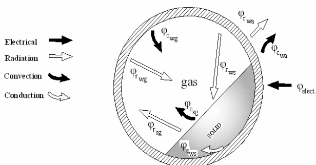
شکل ۵- طرح‌واره‌ای از انواع سازوکارهای انتقال حرارت در رآکتورهای دوار.
