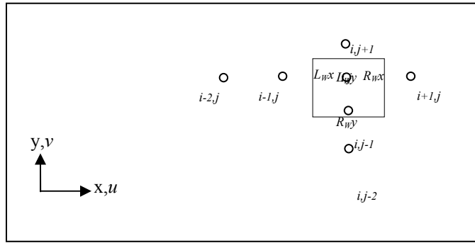
شکل ۳- نقاط مورد استفاده در الگوی منقطع سازی مرتبه دوبرای حالت دو بعدی در پلان
