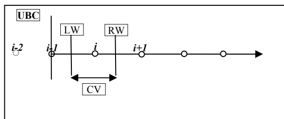
شکل ۲- نقاط مورد استفاده در الگوی منقطع سازی مرتبه دودر نزدیکی مرز بالا دست
