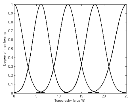
شکل ۴- تابع عضویت توپوگرافی دشت
