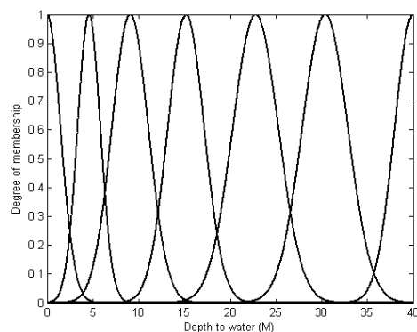
شکل ۲- تابع عضویت عمق سطح آب دشت
