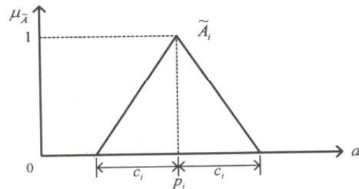
شکل ۴- تابع عضویت ضرائب فازی
