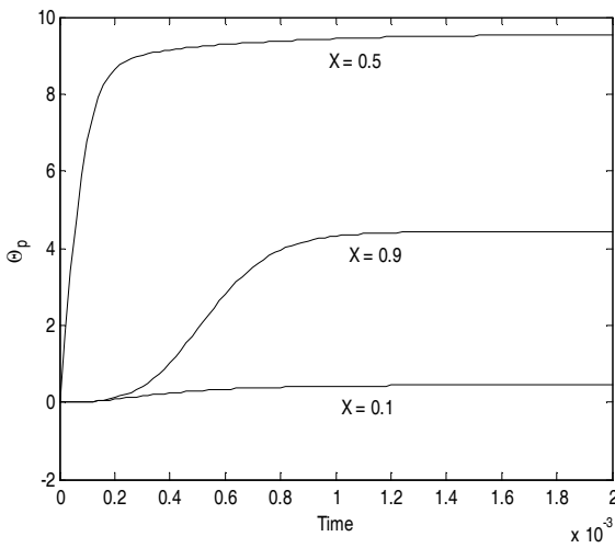
شکل ۵- تغییرات زمانی دما در نقاط مختلف لایه متخلخل
