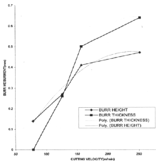
نمودار (۱): نمودار تأثیر پارامتر سرعت برشی بر ابعاد پلیسه.
