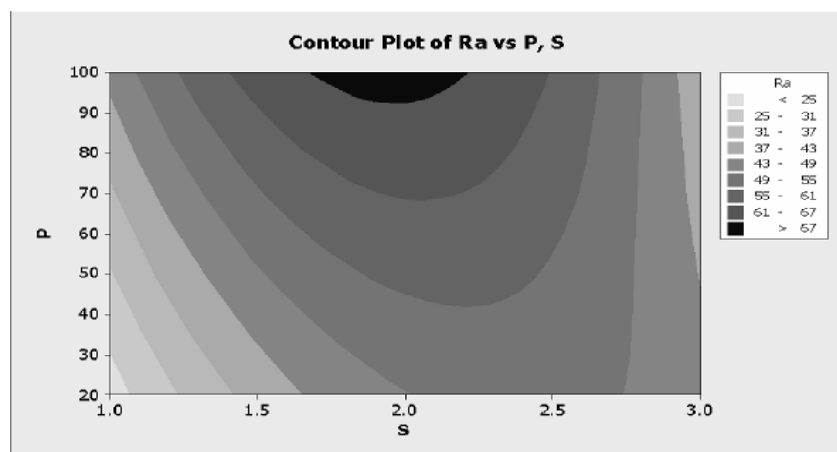
شکل (۶): نمودار کانتوری مربوط به تأثیر دو فاکتور نوع ذره و فشار بر زبری سطح.
