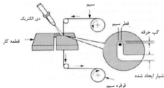
شکل (۱): فرآیند تخلیه الکتریکی سیمی.
