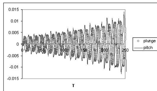
شکل (۱۲): پاسخ زمانی درجات آزادی نوک بال ۴۴۵.۶ مدل توپر در سرعت ۱۴۷ متر بر ثانیه.
