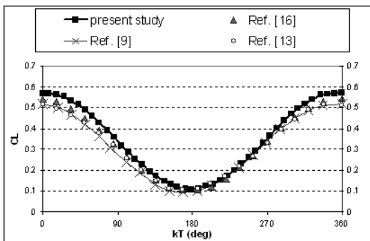
شکل (۵): توزیع ضریب برآ در حرکت نوسانی با فرکانس ۰/۳.
