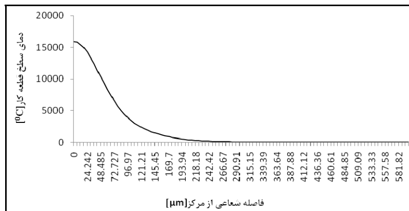
شکل (۴): نمودار تغییرات دما در سطح قطعه‌کار بلافاصله پس از قطع کانال پلازما.
