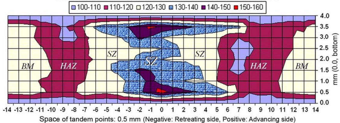
شکل (۱۳): نقشه سختی‌سنجی روبشی مقطع نشان‌داده‌شده در شکل ۶، به روش UCI و تهیه‌شده توسط برنامه اِکسپل.
