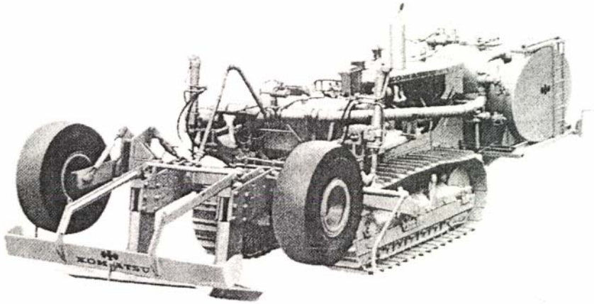
عکس شماره ۱- تراکتور D150-1 ویژه تزریق و پخش لایه غیرقابل نفوذ قیر در زیر شنزار
