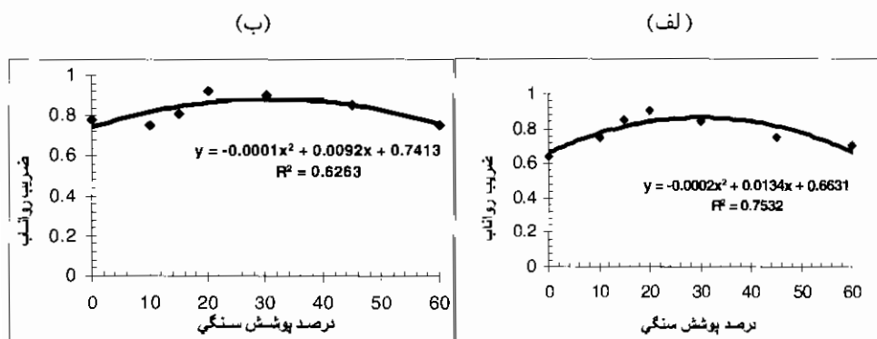
شکل شماره ۵- تغییرات ضریب رواناب با درصدهای مختلف پوشش سنگی (الف) نمونه خاک حوزه ساوه و (ب) نمونه خاک حوزه امامه
