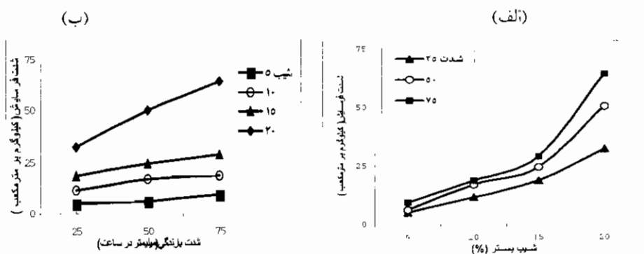
شکل شماره ۱- تأثیر شیب بستر و شدت بارندگی بر روی شدت فرسایش در (الف)
