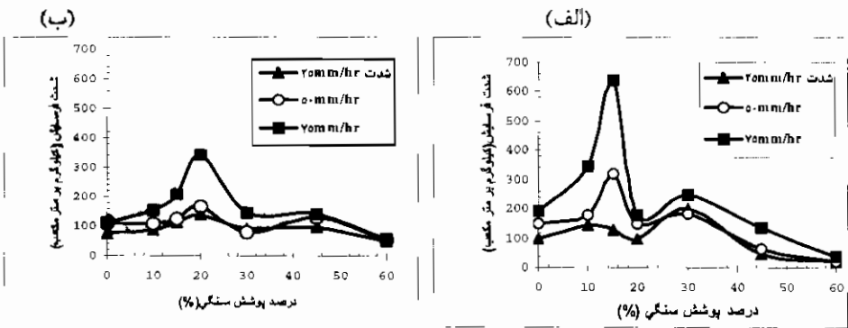
شکل شماره ۲- رابطه بین شدت فرسایش و درصد پوشش سنگی در شدت‌های مختلف با شیب ثابت ۲۰٪ (الف) نمونه خاک حوزه ساوه و (ب) نمونه خاک حوزه امامه
