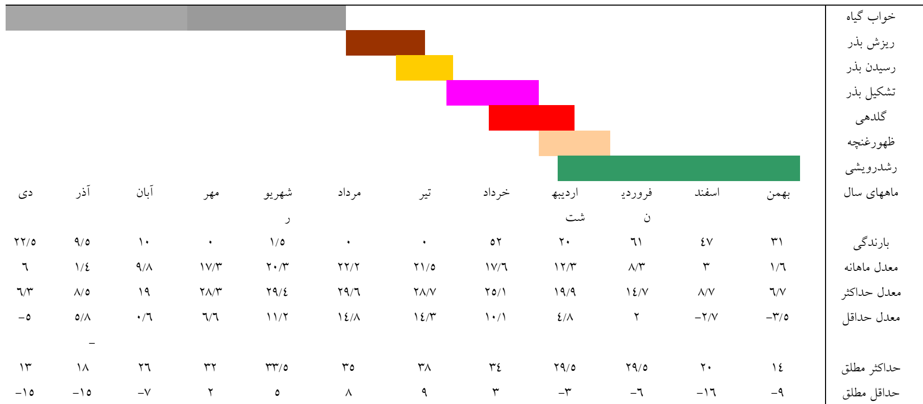
نمودار ۱- نمایش مراحل مختلف فنولوژی Hedysarum kopetdaghi و عوامل مختلف آب و هوایی در رویشگاه سولگرد سال ۱۳۸۱-۱۳۸۲
