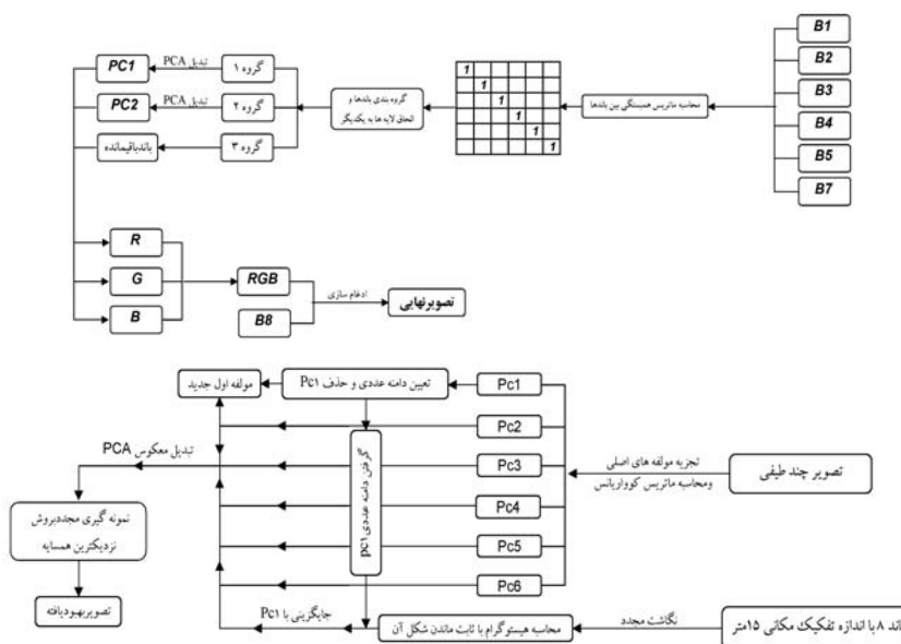
شکل ۴- نمودار جریان مورداستفاده در بارسازی و ادغام داده های ماهواره ای ETM+
