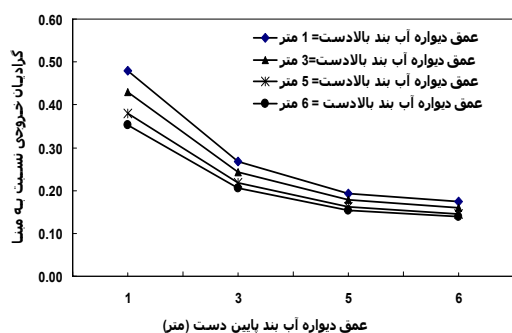
(شکل ۱۳) - مقایسه گرادیان خروجی نسبت به حالت مبنای برای حالت‌های مختلف عمق دو دیواره آب بند
