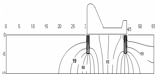
(شکل ۱۱) - خطوط هم پتانسیل ترسیم شده برای حالت دو دیوار آبند هم عمق در بالادست و پائین دست
