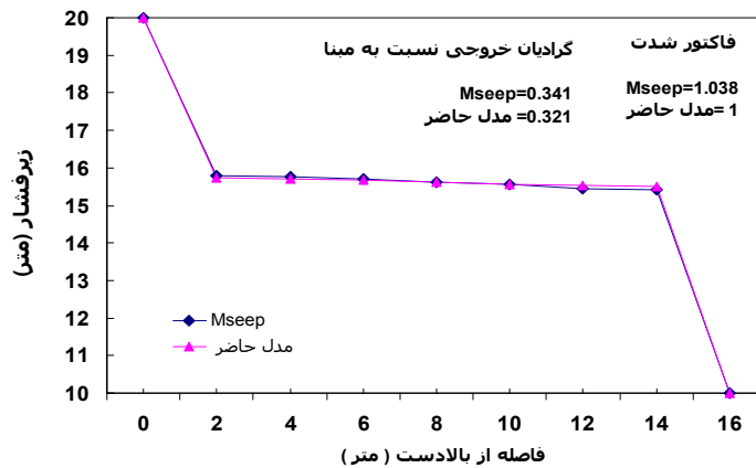
(شکل ۲۳) - مقایسه مقادیر زیرفشار محاسبه شده توسط دو مدل
