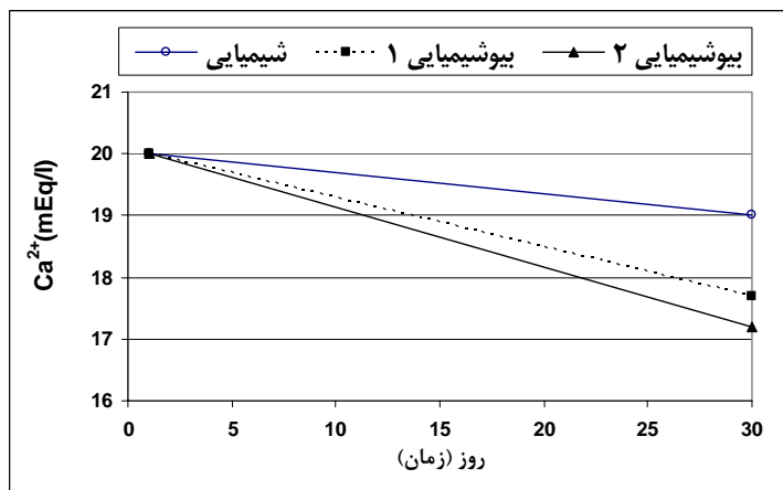
شکل ۵ - روند تغییرات یون کلسیم در طی آزمایش برای تیمارهای بی هواز
