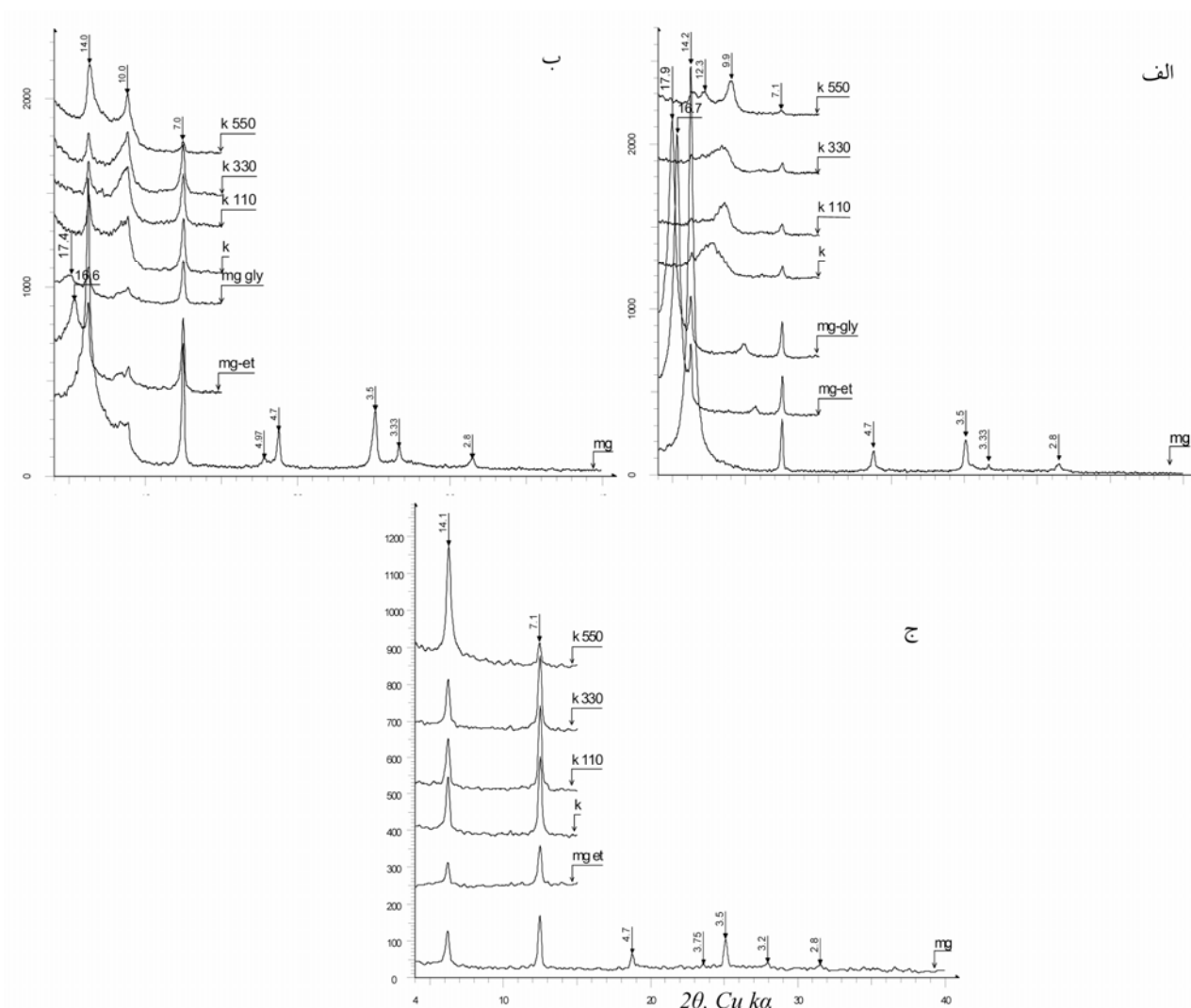
شکل ۲- پراش نگاشت‌های رس سنگ بازالت و خاک حاصل از آن (الف) افق A، (ب) افق BC، (ج) سنگ بازالت. mg: نمونه اشباع با منیزیم، mg-et: نمونه منیزیم اشباع با اتیلن گلیکول، mg-gly: نمونه منیزیم اشباع با گلیسرول، k: k550, k330, k110: به ترتیب، نمونه اشباع با پتاسیم و حرارت‌های ۱۱۰، ۳۳۰ و ۵۵۰ درجه سانتی‌گراد
