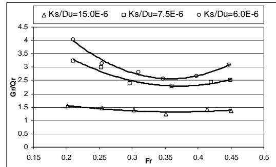
شکل ۳- تغییرات G_r/Q_r بر حسب F_r برای نسبت‌های مختلف K_s/D_u
