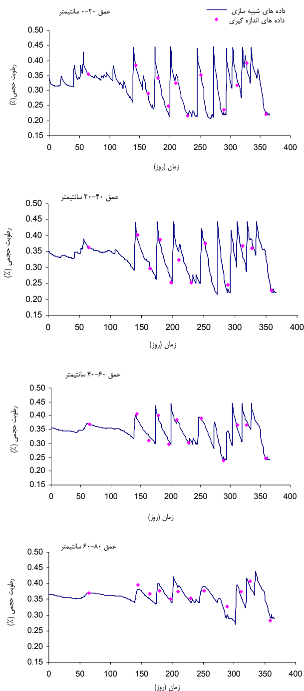
شکل ۳- رطوبت خاک اندازه‌گیری شده و برآورد شده در اعماق مختلف خاک در واحد زراعی A12-3 در سال زراعی ۱۳۸۵-۸۶
