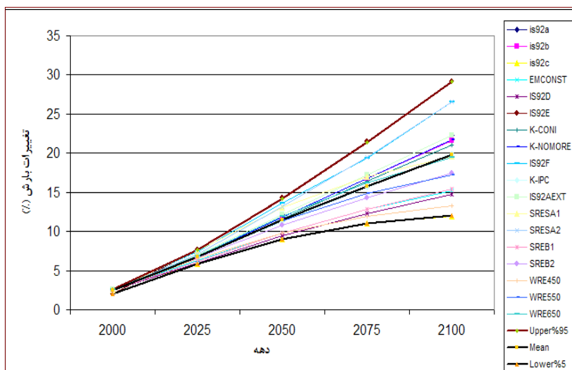
شکل ۴- بر آورد تغییرات دهه ای بارش در دوره ۲۰۰۰-۲۱۰۰ کشور توسط الگو MAGICC SCENGEN با استفاده از داده‌های الگو گردش عمومی جو ECHAM4
