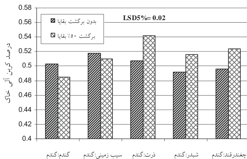
شکل ۲- اثر متقابل تناوب زراعی و برگشت بقایا بر میزان کربن آلی خاک در عمق ۶۰-۳۰ سانتی‌متری خاک در پایان سال دوم آزمایش
