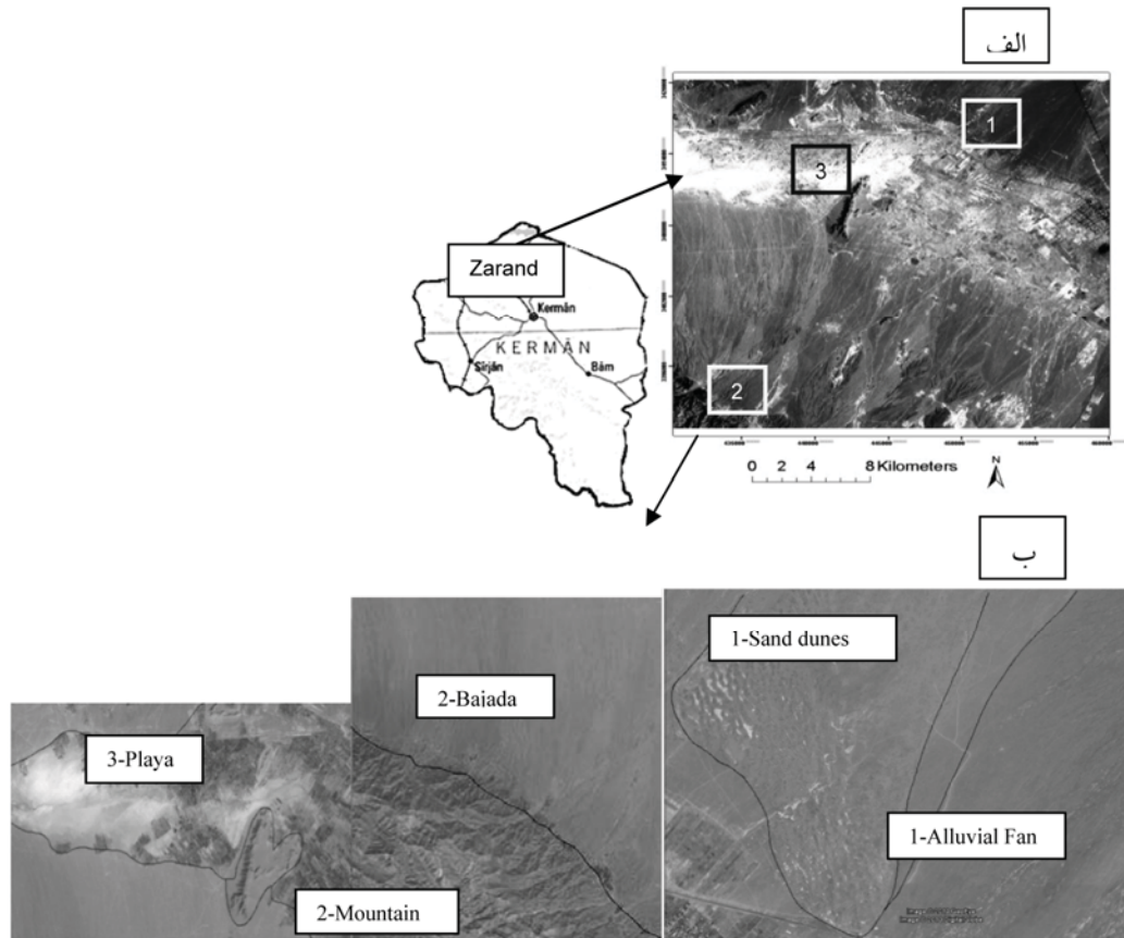
شکل ۱- منطقه مطالعاتی نزدیک شهر کرمان (الف: تصویر ماهواره‌ای لندست ETM (243 RGB)، ب: تصویر تهیه شده توسط Google Earth)
