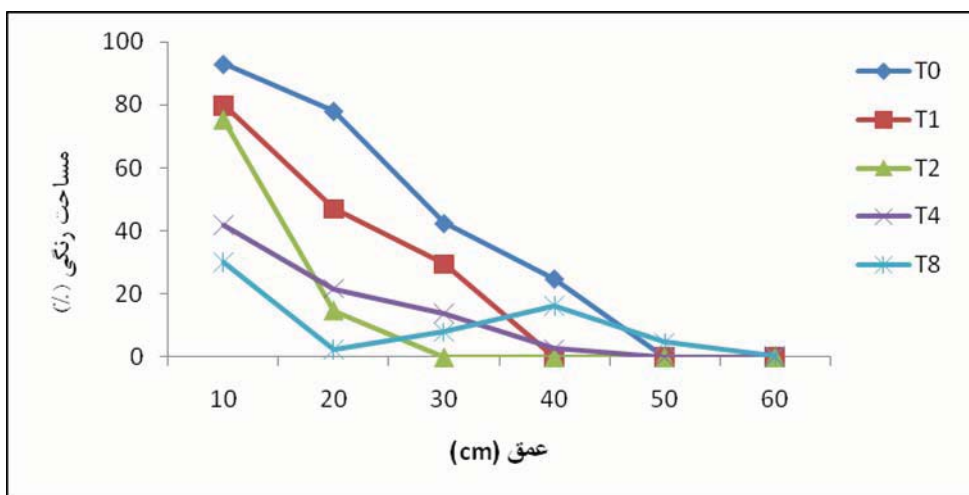
شکل ۶- درصد مساحت رنگی عمق‌های مختلف تیمارهای مورد آزمایش (اندیس‌ها بیان کننده تعداد عبور تراکتور می‌باشند)
