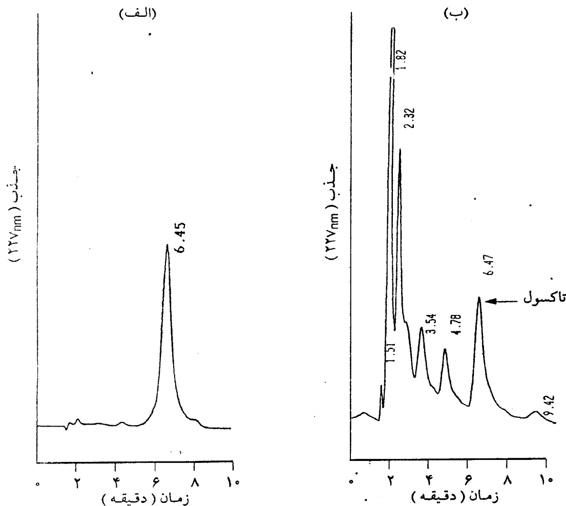
شکل ۱- کروماتوگرام‌های مربوط به استاندارد تاکسول (الف) و عصاره کالوس‌های بدست آمده از جداکشت‌های برگ سرخدار (ب)
