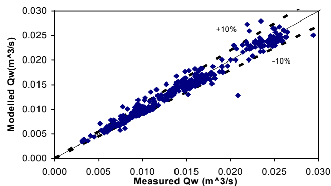
شکل ۵. مقایسه دبی سرریز اندازه گیری شده و محاسبه شده در آزمونها بدون در نظر گرفتن عامل منشوری و کنترل
