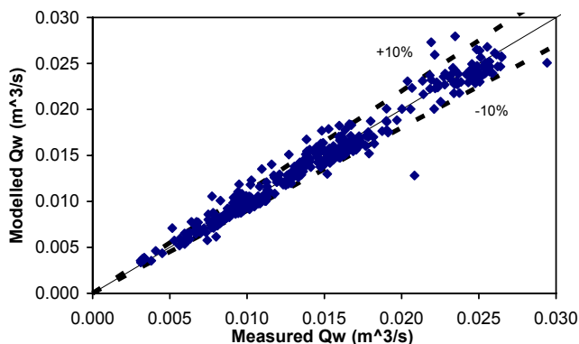
شکل ۴. مقایسه دبی سرریز اندازه گیری شده و محاسبه شده در آزمونهای با کنترل در پایین دست
