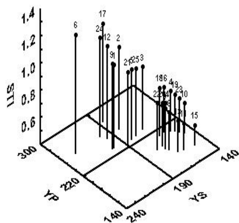
شکل ۴- نمودار تعیین ژنوتیپ‌های متحمل به خشکی بر اساس شاخص STI در ژنوتیپ‌های نخود Ys: عملکرد بالقوه هر ژنوتیپ تحت شرایط تنش محیطی، Yp: عملکرد بالقوه هر ژنوتیپ تحت شرایط مطلوب و SSI: شاخص تحمل تنش. اعداد روی هر میله شماره ژنوتیپ مربوطه می‌باشد.
