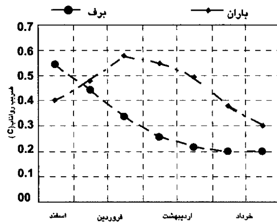
شکل ۳ - نمودار تغییرات ضریب رواناب برف و باران
