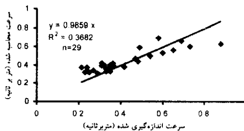
شکل ۱۱- مقایسه سرعت اندازه گیری شده و محاسبه شده با معادلات سیمونز و آلبرستون.
