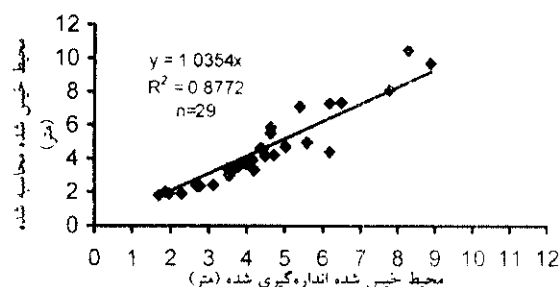
شکل ۴- مقایسه مقادیر محیط خیس شده اندازه‌گیری شده و محاسبه شده با استفاده از معادلات سیمونز-آلبرستون.
