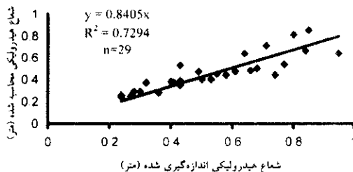
شکل ۷- مقایسه شعاع هیدرولیکی اندازه گیری شده و محاسبه شده با معادلات سیمونز و آلبرستون.
