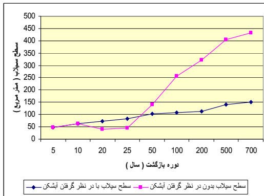
شکل ۴- مقایسه عمق (راست) و سطح سیلاب (چپ) در بازه با آب شکن ۱ و بدون آن.
