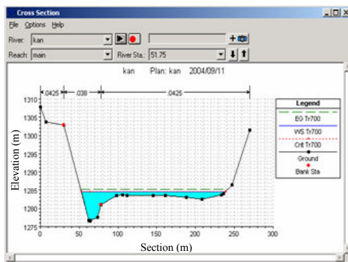
شکل ۵- وضعیت سطح آب در دبی با دوره بازگشت ۷۰۰ ساله در صورت
