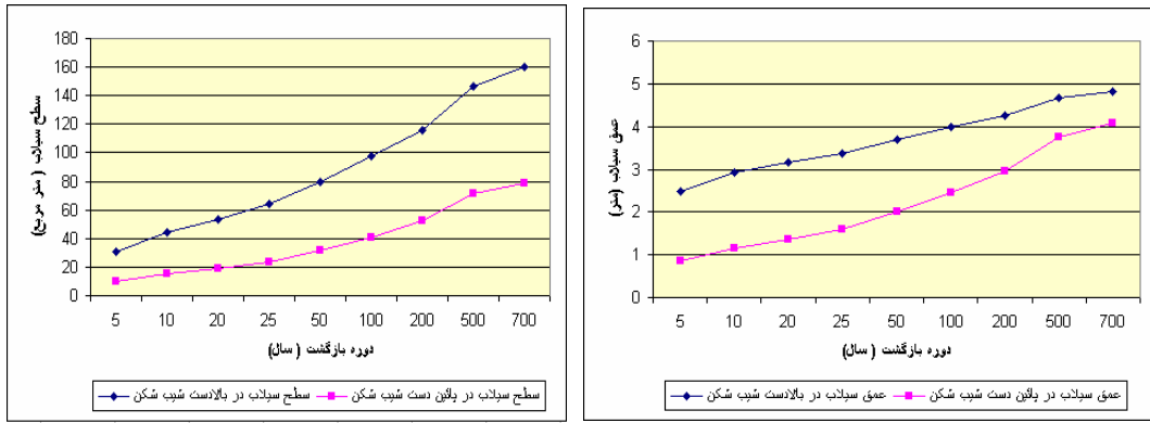
شکل ۹- مقایسه عمق سیلاب (راست) و سطح سیلاب (چپ) در بالادست و پائین دست شیب شکن ۱.
