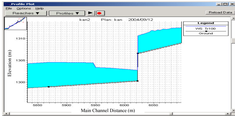
شکل ۱۱- نمای پروفیل جریان در محل شیب شکن ۲.
