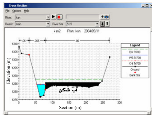
شکل ۵- وضعیت سطح آب در دبی با دوره بازگشت ۷۰۰ ساله در صورت
