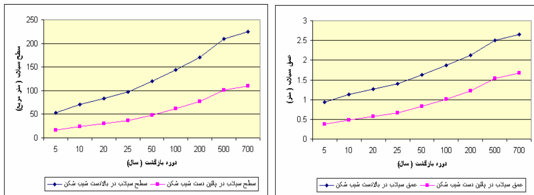
شکل ۱۲- مقایسه عمق سیلاب (راست) و سطح سیلاب (چپ) در بالادست و پائین دست شیب شیکن ۲.
