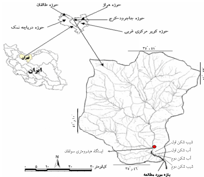
شکل ۱- سیمای کلی حوزه آبخیز کن و بازه مورد مطالعه
