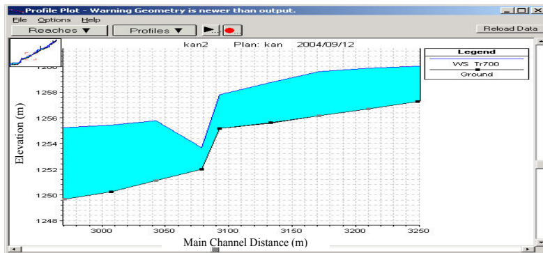
شکل ۷- نمای پروفیل جریان در محل شیب شکن ۱.
