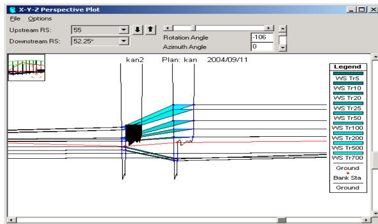
شکل ۲- نمای وضعیت جریان با دوره‌های بازگشت مختلف در آب شکن ۱.
