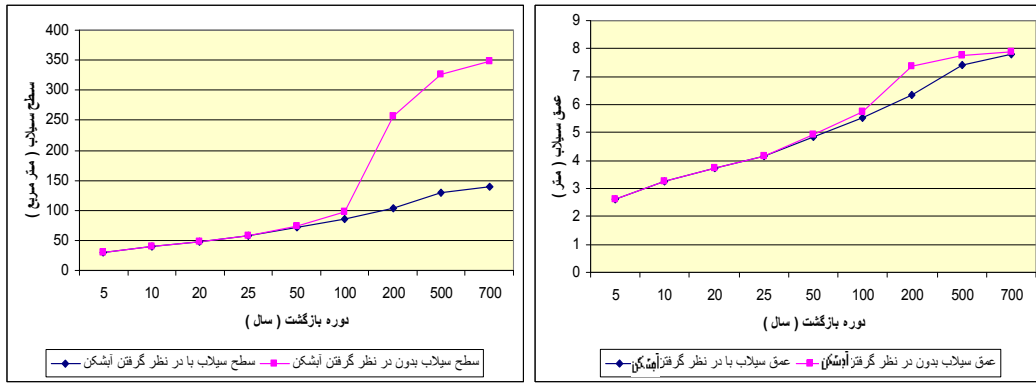
شکل ۶- مقایسه عمق (راست) و سطح سیلاب (چپ) در بازه با آب شکن ۲ و بدون آن.
