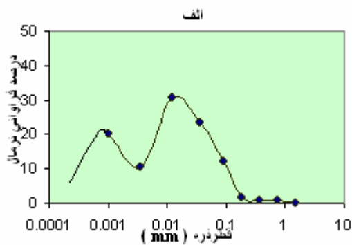
شکل ۲- نمودارهای نرمال (الف) و تجمعی (ب) توزیع اندازه ذرات مقطع قیان (افق Ck3).
