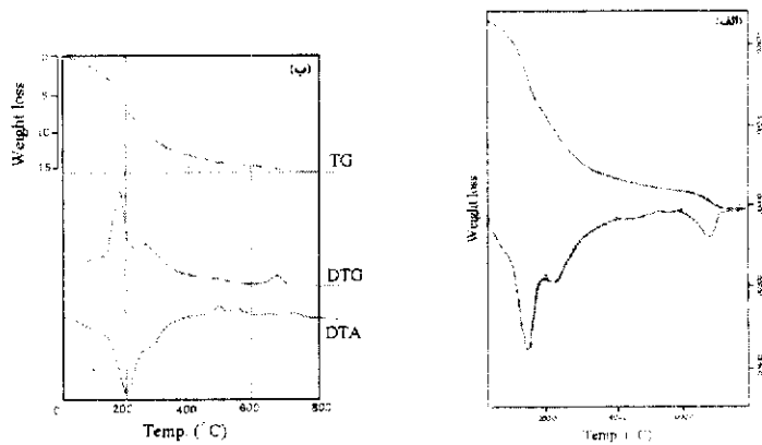
شکل ۳ منحنی‌های گرمایی (الف) نمونه منطقه طالقان، (ب) نمونه مرجع [۱]
