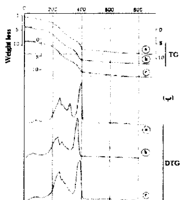
شکل ۲ منحنی‌های گرمایی (الف) نمونه گردنه ملا احمد، (ب) نمونه مرجع [۱].
