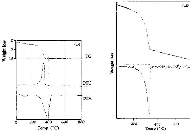
شکل ۱ منحنی‌های گرمایی (الف) نمونه جنوب تهران، (ب) نمونه مرجع [۱].
