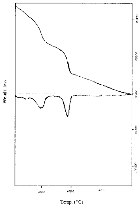
شکل ۵ نحی گرمای (TG,DTG) نمونه منطقه کرکس
