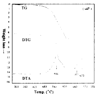
شکل ۲ منحنی‌های گرمایی (الف) نمونه گردنه ملا احمد، (ب) نمونه مرجع [۱].
