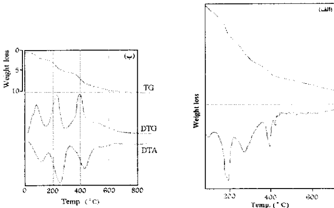
شکل ۴ منحنی‌های گرمایی (الف) نمونه قلعه خرگوشی (ب) نمونه مرجع [۱].
