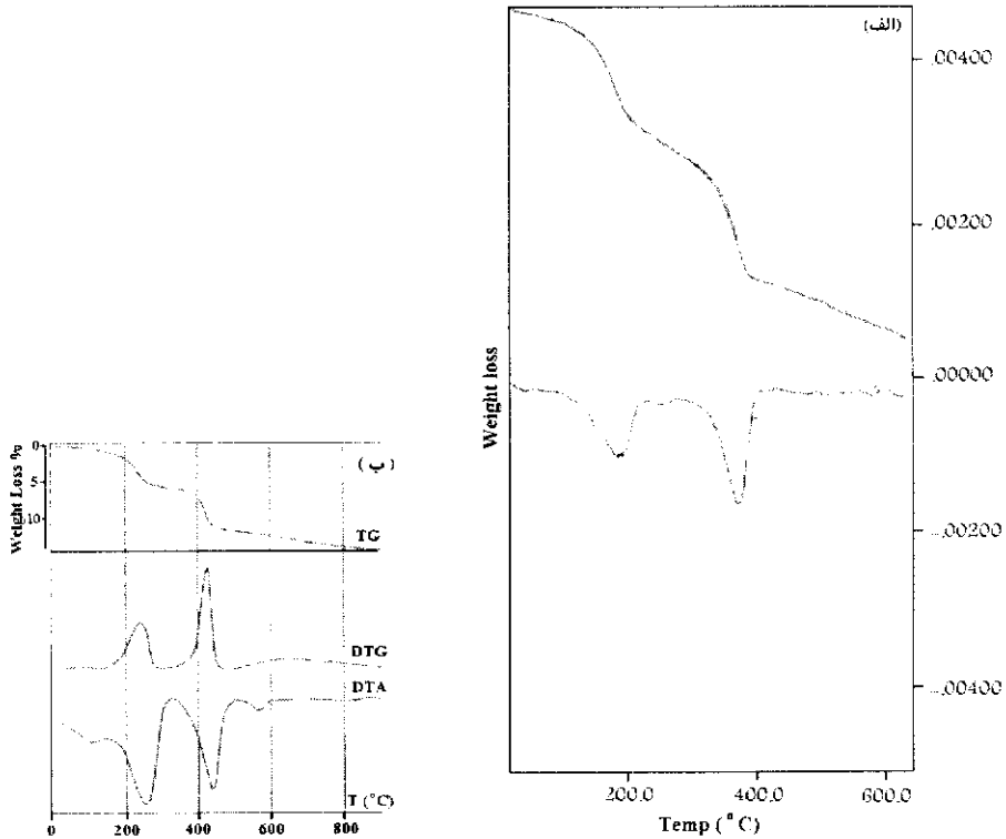
شکل ۱۰ منحنی‌های گرمایی (الف) نمونه منطقه اردستان، (ب) نمونه مرجع [۲].
