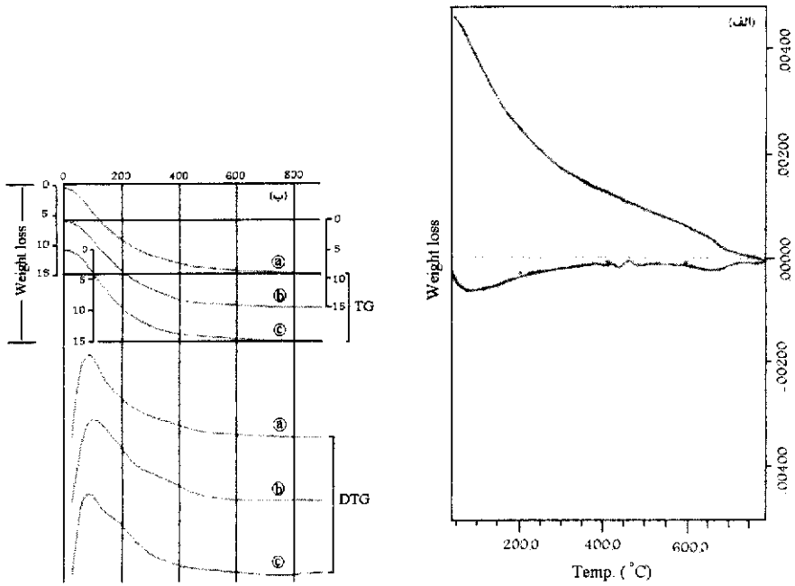
شکل ۸ منحنی‌های گرمایی (الف) نمونه منطقه سمان، (ب) نمونه مرجع [۱].
