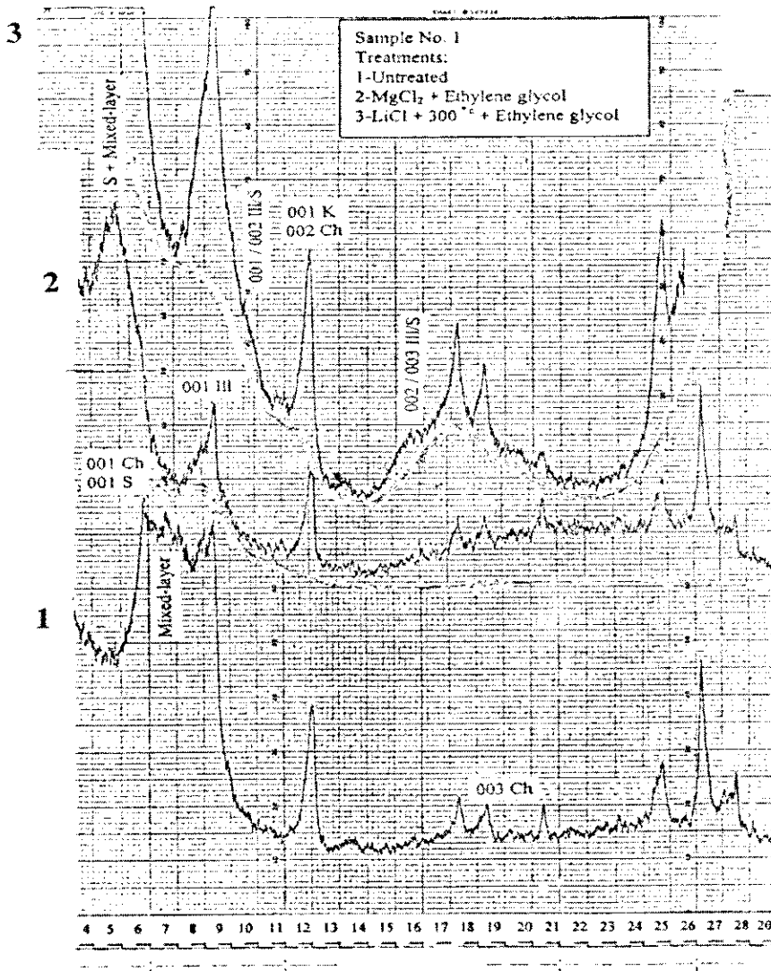
شکل ۱ نمودار پرتو ایکس از یک درهم کانی رسی که بخش اصلی آن را درهم لایه نامنظم ایلیت - اسمکتیت تشکیل داده است. سه تیمار نمونه خام، کلرید منیزیم و کلرید لیتیوم در شکل با شماره مشخص شده‌اند (لامپ مس).
