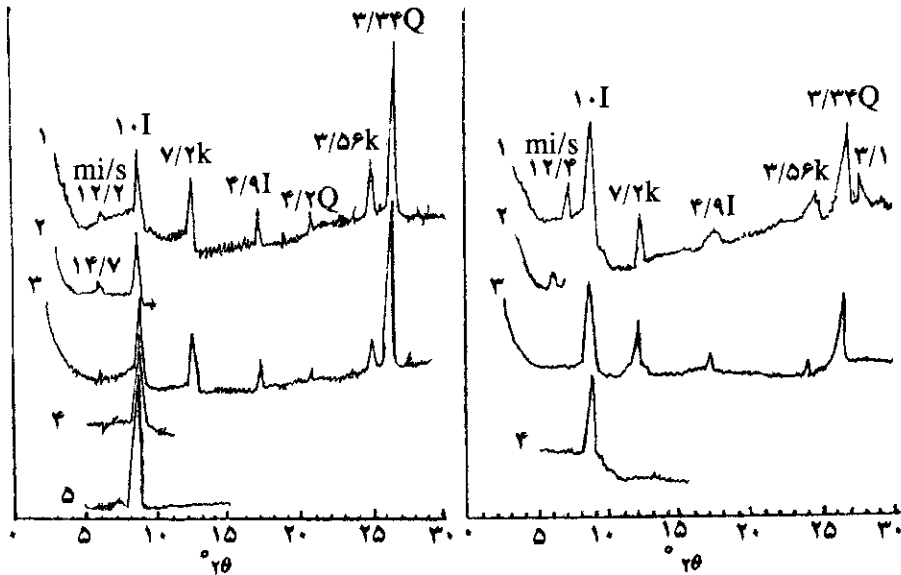
شکل ۷ پراش نگاشت پرتو ایکس ذرات رس
