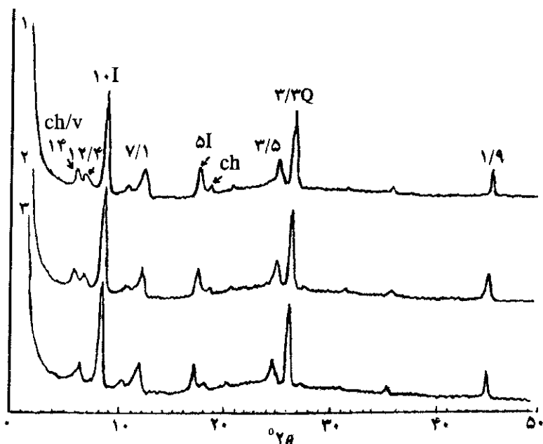
شکل ۳ پراش نگاشت پرتو ایکس از ذرات رس سنگ فیلایت هوازده (نیمرخ خاک ۱) پراش نگاشت ۱: نمونه اشباع شده با منیزیم. پراش نگاشت ۲: نمونه ۱ + گلیکول. پراش نگاشت ۳: نمونه اشباع با پتاسیم + دمای 550^{\circ}\text{C} به مدت ۲ ساعت.
