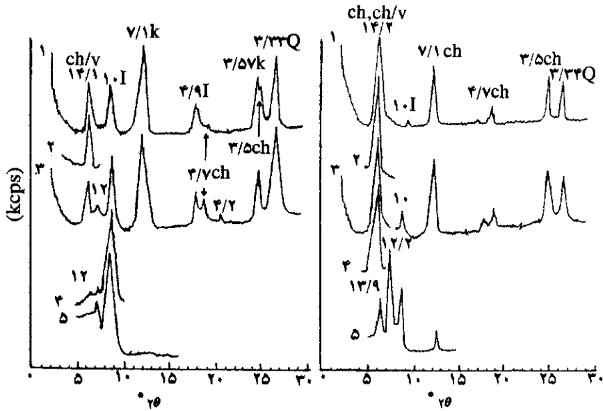
شکل ۲ پراش نگاشت پرتو ایکس ذرات رس افق C (۱۷۵-۱۲۲، نیمرخ خاک ۱).
