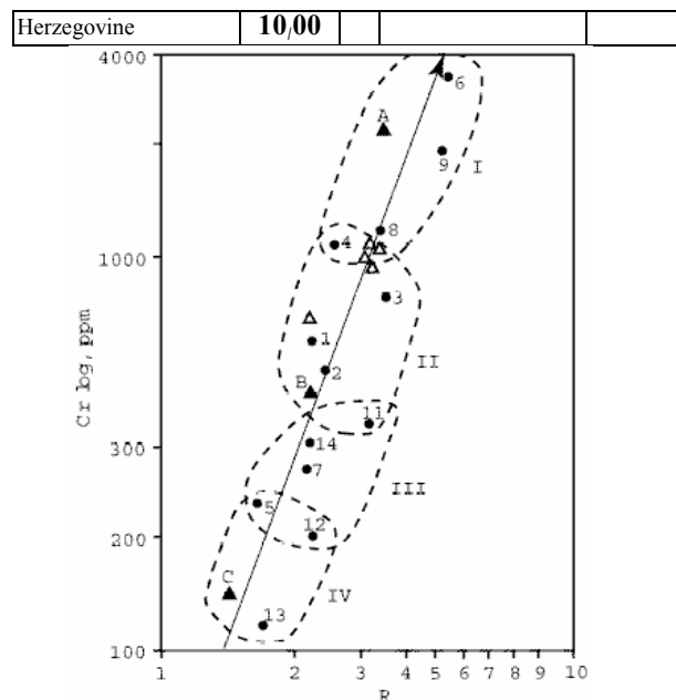
شکل 5 تغییرات ضریب انباشتگی (R) عناصر کمیاب در نمونه‌های بوکسیت قپی (مثلث‌های تو خالی) و مقایسه آن با بوکسیت‌های کارستی مدیترانه ای و لاتریتی ارکانزاس به عنوان تابعی از عنصر Cr [10]. I, II, III, IV به ترتیب بیانگر مناطق اثر سنگهای مادر الترامافیک، مافیک، حد واسط و اسیدی هستند. B, A و C (مثلث‌های توپر) به ترتیب مربوط به لاتریت‌های حاصل از آمفیبولیت، بازالت و گرانیت هستند. برای توضیح اعداد به شکل 4 مراجعه کنید.
