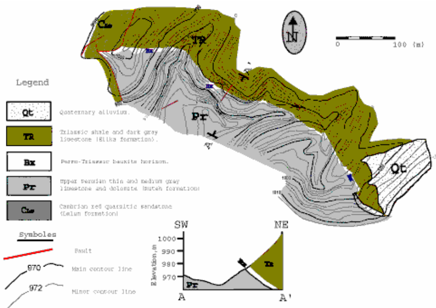
شکل 1 نقشه زمین‌شناسی منطقه مورد مطالعه [1].
