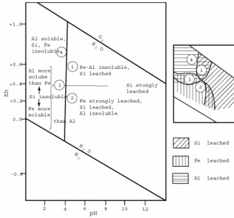
شکل 7 نقش pH و Eh در تشکیل بوکسیت‌ها با توجه به تحرک عناصر [18].
