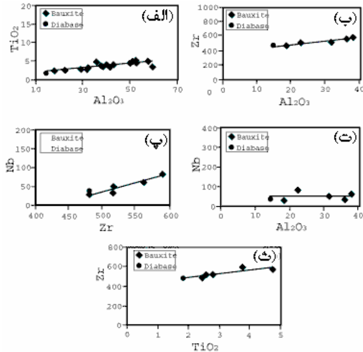
شکل 6 نمودارهای همبستگی، الف) Al_2O_3 - TiO_2 ، ب) Al_2O_3 - Zr ، پ) Zr - Nb ، ت) Al_2O_3 - Nb ، ث) TiO_2 - Zr نمونه های بوکسیتی و سنگ دیاباز [15]. خط پیوسته حاصل از درون یابی بهترین خط روند هوازدگی است.
