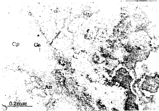
شکل ۵ کالکوپیریت (Cp) بفرم جزیره مانند درون محصولات اکسیداسیون و هوازده، گیریت (Ge) در اطراف کالکوپیریت و آنیلیت (An) بصورت تیغه‌های تقریباً موازی دیده می‌شود.
