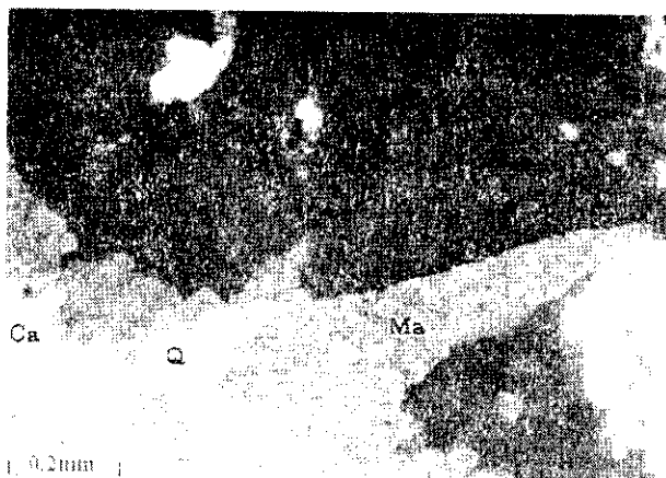
شکل ۱۰ خنثی شدن محلولهای اسیدی مس دار حاصل از هوازدگی کالکوپیریت، توسط کانیهای کربناته سنگ میزبان و شکل گیری ملاکیت (Ma).
