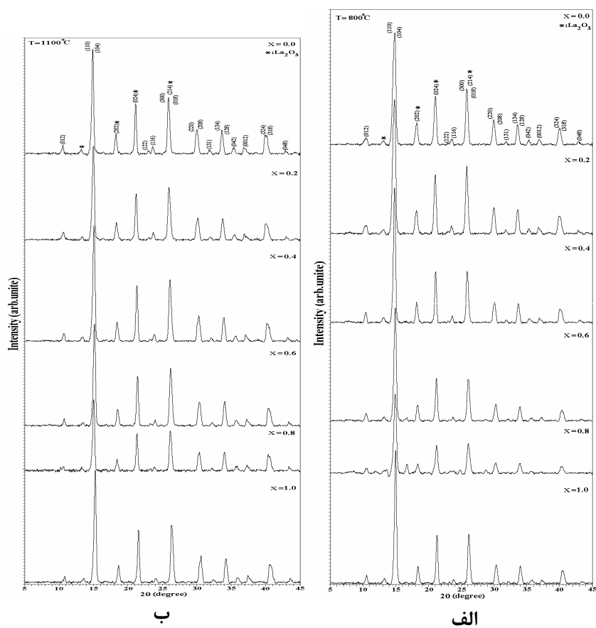
شکل ۲ الگوهای پراش پرتو X ( \lambda = 0.7093 ) ترکیب \text{La}_{0.75}\text{Sr}_{0.25}\text{Mn}_{1-x}\text{Co}_x\text{O}_3 به ازای مقادیر مختلف X، پس از خشکاندن در دمای 400^\circ\text{C} .
