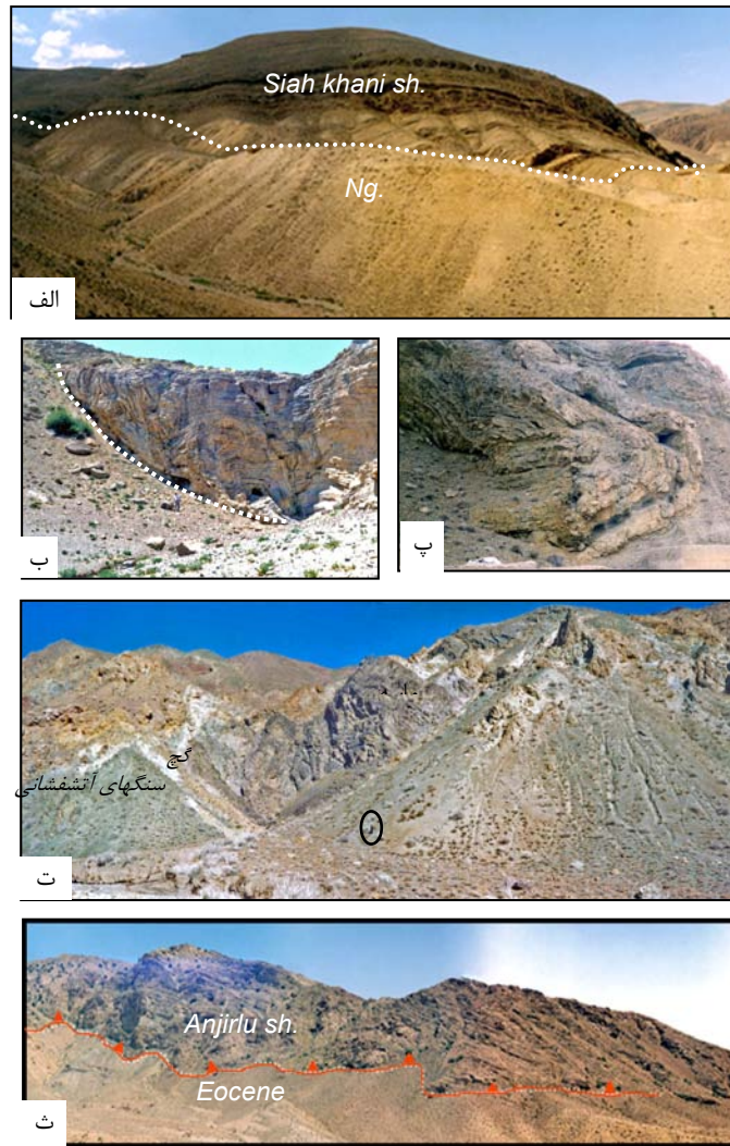
شکل ۲ الف) قاعده برگه راندگی سیاه‌خانی در شمال روستای توبه‌رودبار، سازند مبارک به سوی جنوب‌شرق روی دنباله‌های نئوژن رانده شده است. دید به سمت شمال. ب) چین فرادیواره‌ای برگه راندگی سیاه‌خانی در شمال روستای توبه، دید به سمت شمال‌شرق. پ) راندگی فرعی درون برگه راندگی سیاه‌خانی در شمال روستای توبه، دید به سمت غرب. ت) بخش خرد شده در فرودیواره برگه طزره، دره تالو در شمال‌شرق دامغان، دید به سمت N005. به جایگزینی به صورت برگه سنگهای آتشفشانی بازیک، گچ، شیل، و ماسه‌سنگهای سبز زیتونی روی هم توجه فرمایید. ث) قاعده دوتایی میانی انجیرلو که به وسیله آن طبقات پالئوزوییک روی ائوسن شیربند رانده شده است. جاده چشمه‌علی، شمال غرب دامغان، دید به سمت جنوب‌شرق.
