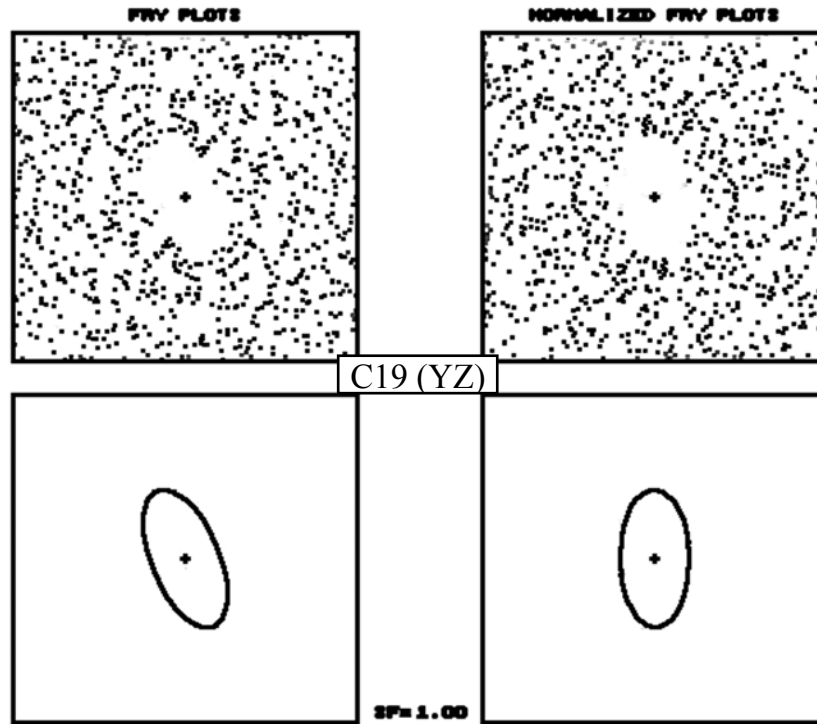
شکل ۸. نمونه‌هایی از محاسبه بیضویهای تنش نهایی با دو روش Fry و بهنجار Fry با نرم‌افزار Instrain (Erslev, 1988).
