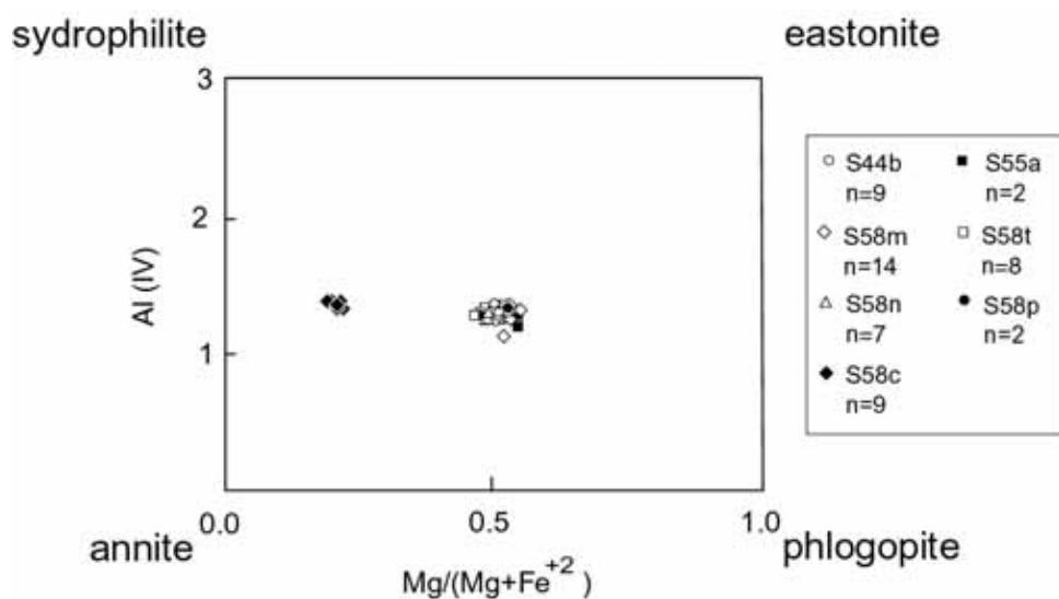
شکل ۲ توزیع ترکیب بیوتیت‌های آنالیز شده از شیستهای SMC. بجز یک نمونه، ترکیب بقیه بیوتیتها مشابه است.
