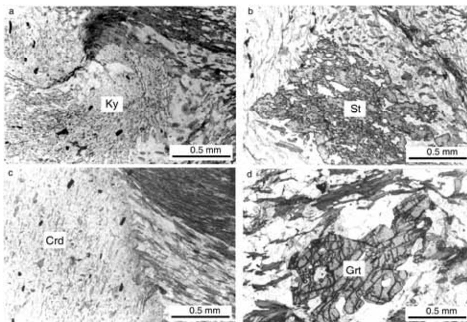
شکل ۲ تصاویر میکروسکوپی در حالت PPL از میکاشیستهای دگرگون به صورت ناحیه ای. a درشت بلور کیانیت. b ایدیوبلاست استارولیت با ماکل صلیبی. c پورفیروبلاست کردیریت با بافت پوئیکلیتیک. d پورفیروبلاست گارنت.
