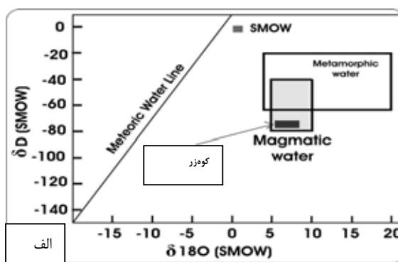
شکل ۸ الف بر پایه نمودار [۲۳] ترکیب ایزوتوپی شاره‌های گرمابی کانی‌سازی در گستره آبهای ماگمایی قرار می‌گیرد. با توجه به نمودار (ب) [۲۴] ترکیب ایزوتوپی گوگرد ( \delta^{34}S ) نمونه‌ها نیز نشان‌دهنده ریشه ماگمایی است.
