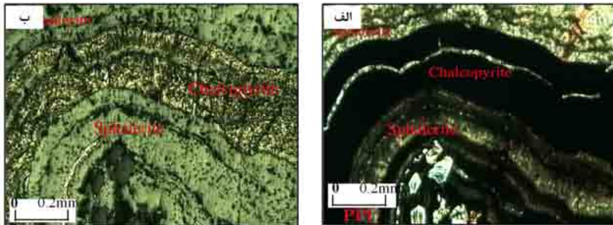
شکل ۷ بافت کلوform (ریتمیک) از کانی اسفالریت در نور PPL عبوری در الف و نور بازتابی در ب.
