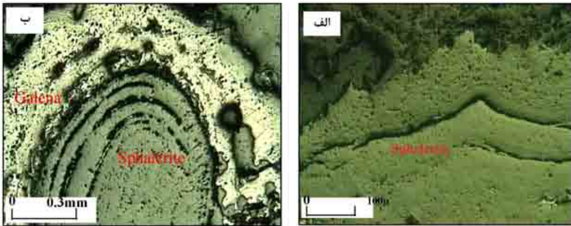
شکل ۸ در الف بافت زونی از کانی اسفالریت و در ب بافت گل کلمی از کانی اسفالریت همراه با گالن.
