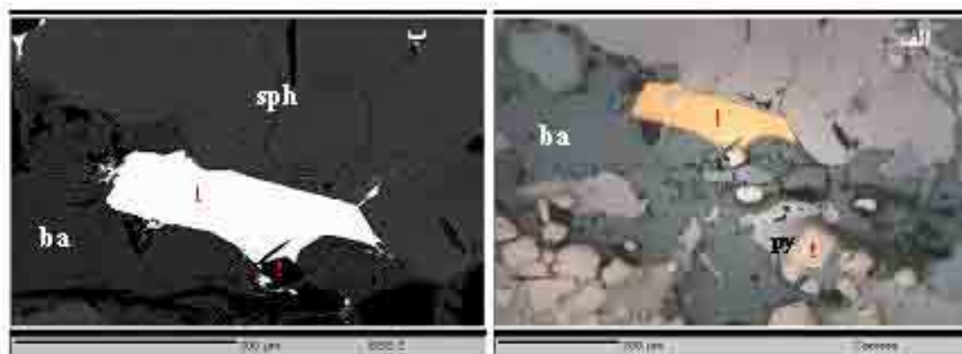
شکل ۳ الف) مهاجرت الکتروم (el) از درون شکستگی پیریت به فضای بین بلورهای باریت (ba) و ب) فرارگیری الکتروم در فضای بین بلور شکسته پیریت.
