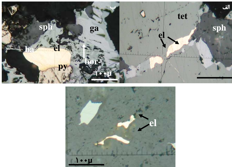
شکل ۵ الف) دو ذره الکتروم (el) موجود در شکستگی تتراندريت (tet) همراه با اسفالريت (sph)، ب) الکتروم درشت و باز تبلور در فضای بین بلورهای پیریت (py)، بورنونیت- بولانتریت (bor-bol)، باریت (ba)، اسفالريت (sph) و گالن (ga)، و ج) دو ذره درشت الکتروم در بلور باریت (ba).
