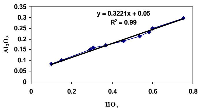
شکل ۱۱ نمودار Al 2 O 3 بر حسب TiO 2 .
