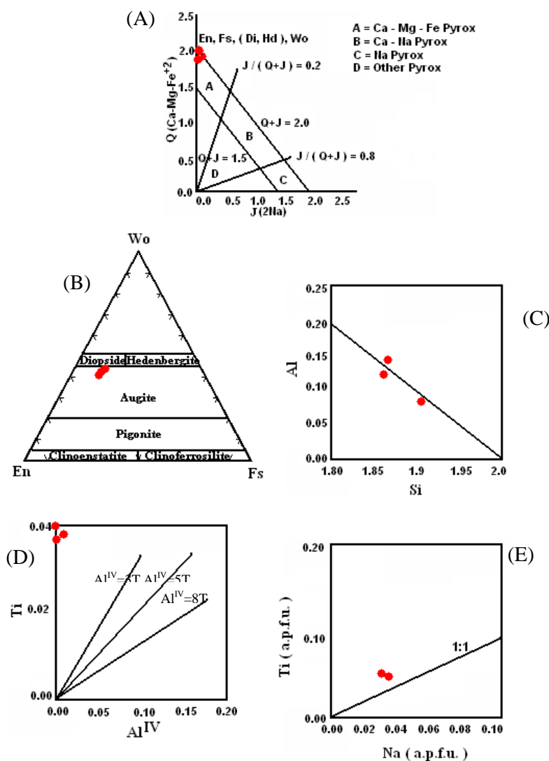
شکل ۳ (A) ترکیب کلینوپیروکسن‌های منطقه [V]، (B) کلینوپیروکسن‌های منطقه روی نمودار مثلثی انستاتیت (En)، ولاستونیت (Wo) و فروسیلیت (Fs)، (C) نمودار Al-Si که نشان دهنده مقدار بالای تیتانیم در این کانی‌ها است، (D, E) نمودارهای Na, Al^{IV} در مقابل Ti.
