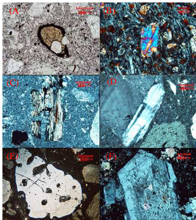
شکل ۲ (A) هورنبلند بازالتی در آندزیت (PPL, 10X)، (B) بلور پیروکسن در آندزی بازالت (XPL, 20X)، (C) نمای از یک بلور فلوگوپیت با میانبار زیرکن (XPL, 10X)، (D) کانی‌های پلاژیوکلاز، ارتوز و کوارتز در ریولیت (XPL, 40X)، (E) کوارتز خلیجی در ریولیت (XPL, 20X)، (F) بافت غربالی در پلاژیوکلاز (XPL, 40X).
