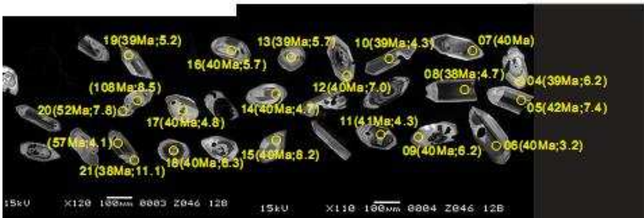
شکل ۹ تصویر CL (کاتد لومینسانس [درخشان]) از ۵۷ دانه زیرکن که در قالب مخصوص قرار داده شده و تعداد ۲۰ دانه‌ی مورد سال سنجی قرار گرفته است. نتیجه حاصل برای هر دانه روی آن نوشته شده است.
