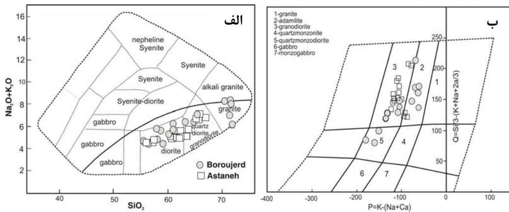
شکل ۲ الف) نمودار \text{SiO}_2 نسبت به مجموع قلیایی [۱۲]، خط جدا کننده گستره قلیایی از آهکی - قلیایی به نقل از [۱۴] ب) رده بندی [۱۳].
