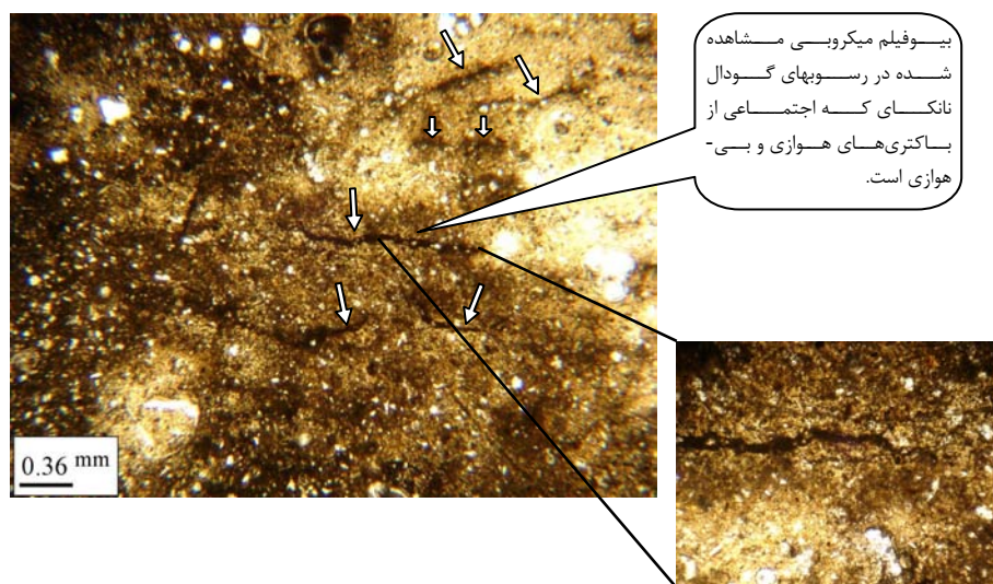
شکل ۵ تصویر میکروسکوپی از بیوفیلم موجود در رسوبهای فرورفتگی نانکای (ppl). پیکان‌ها نشان دهنده‌ی بیوفیلم‌های میکروبی است که به شکل خطوط تیره‌ی، نامنظم و پراکنده قابل مشاهده‌اند. زمینه آلی باکتری‌ها در تشکیل این بیوفیلم‌ها اهمیت فراوانی دارد. زمینه آلی به صورت هاله‌ی شفاف پیرامون باکتری‌های احیا کننده سولفات در شکل ۷ به خوبی دیده می‌شود.
